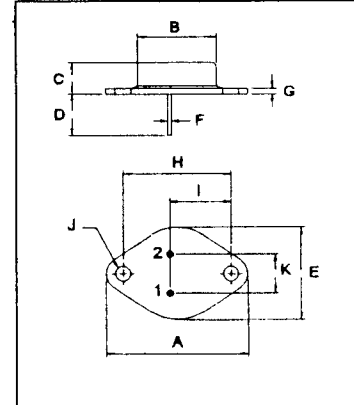
TO-3
